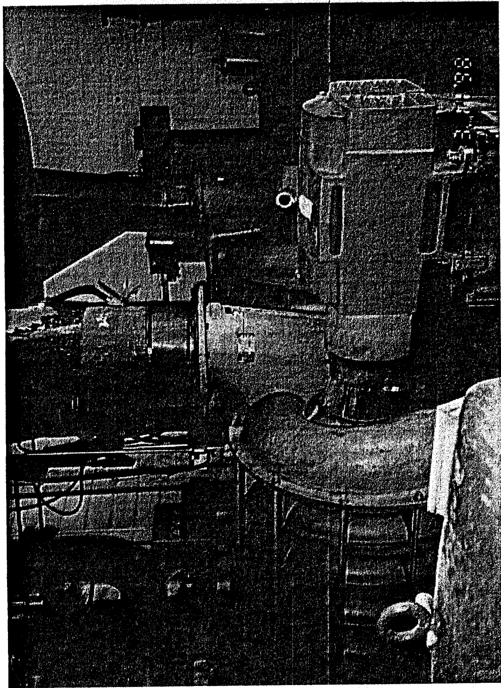
صورة رقم (٥) : مراوح الشفط شفط الهواء متصلة بالمحرك الكهربائي (عالم ديزني - أورلاندو، ١٩٩٨م).
